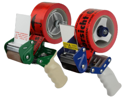
Handabroller T251 für 50 mm Bandbreite.
