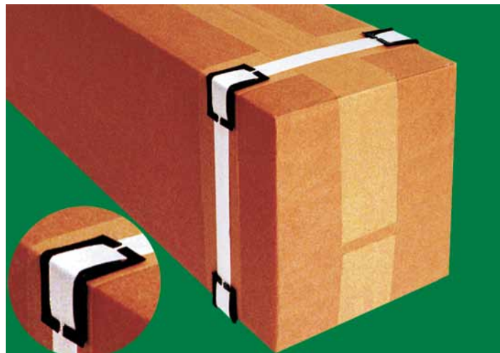
Kantenschutzecken mit Führungsschlitz
