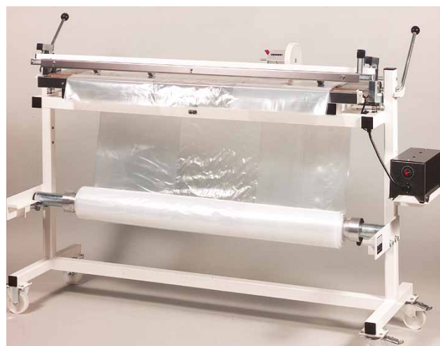
Folienschweißgerät 1500 MS-3 zur Herstellung von Palettenhäuben, mit Längenzähler
